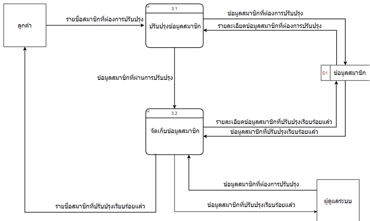
ภาพที่ 3.6 แสดง Data Flow Diagram Level 1 ของการจัดการข้อมูลสมาชิก
