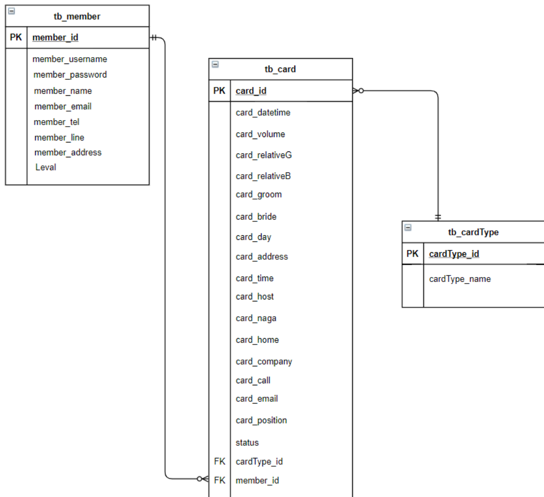
ภาพที่ 3.8 แสดง Entity Relationship Diagram (ERD) ของระบบการจัดการโรงพิมพ์ (ตักฟ้าการพิมพ์)
