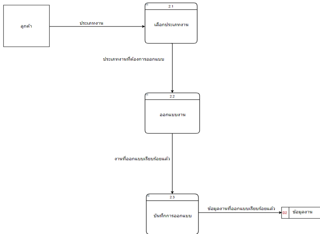
ภาพที่ 3.5 แสดง Data Flow Diagram Level 1 ของการออกแบบงาน
