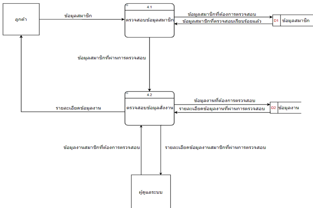
ภาพที่ 3.7 แสดง Data Flow Diagram Level 1 ของการตรวจสอบประวัติการสั่งงาน
