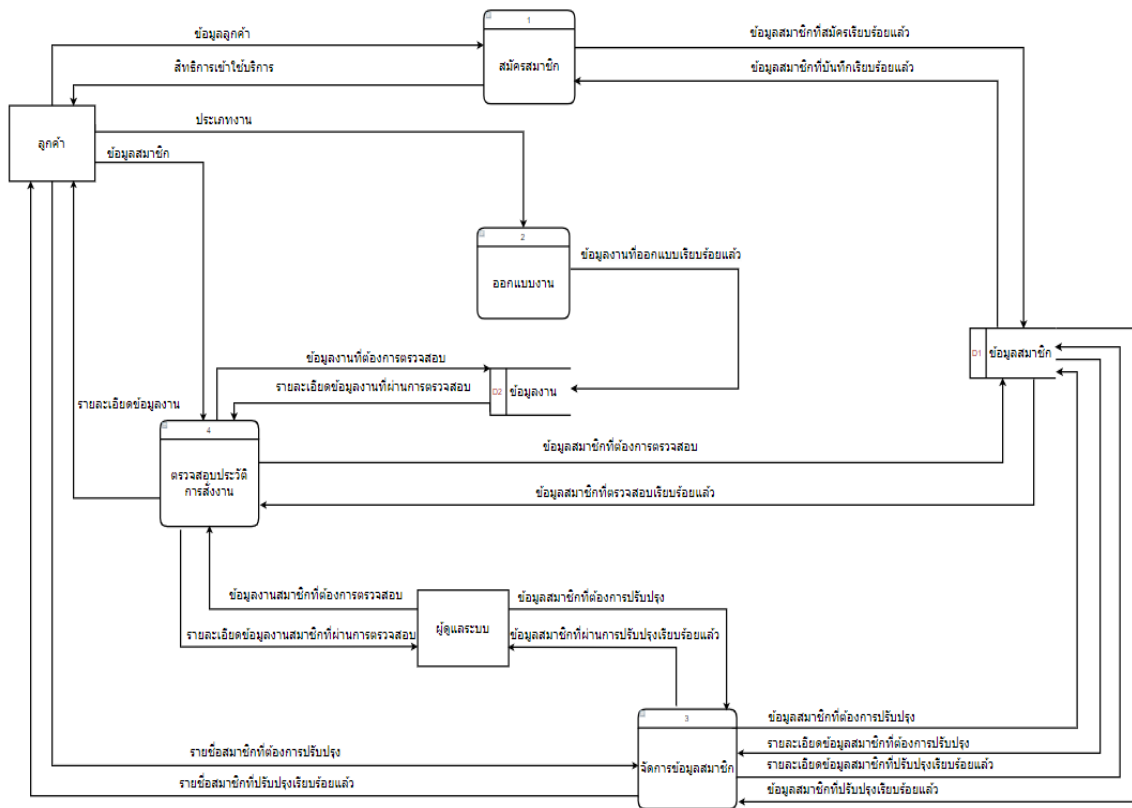
ภาพที่ 3.3 แสดงภาพรวม (Data Flow Diagram Level 0) ของระบบการจัดการโรงพิมพ์ (ตากฟ้าการพิมพ์)
