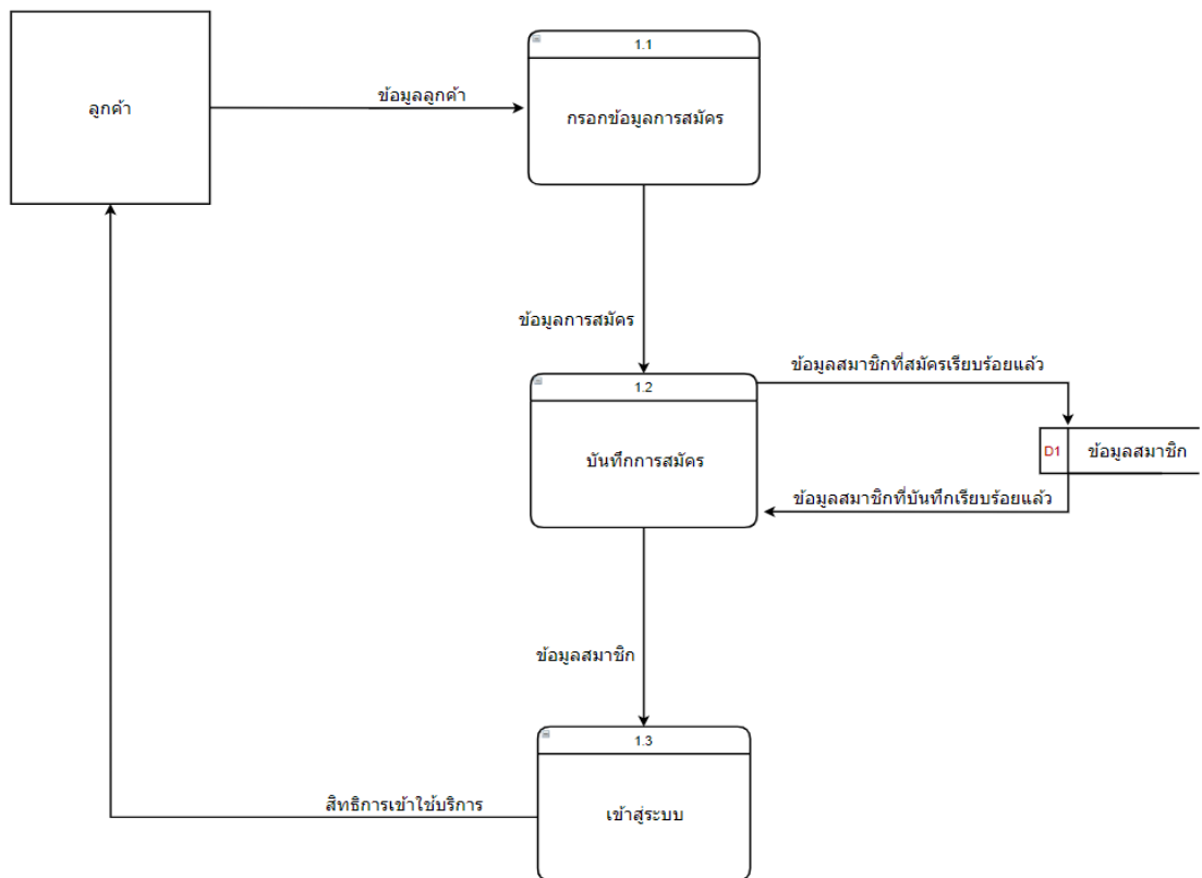
ภาพที่ 3.4 แสดง Data Flow Diagram Level 1 ของการสมัครสมาชิก
